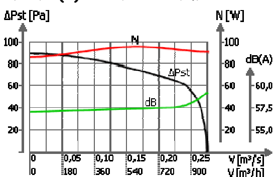
WVPKH(V)-200 /700obr/min
