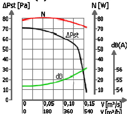
WVPKH(V)-160 /700obr/min
