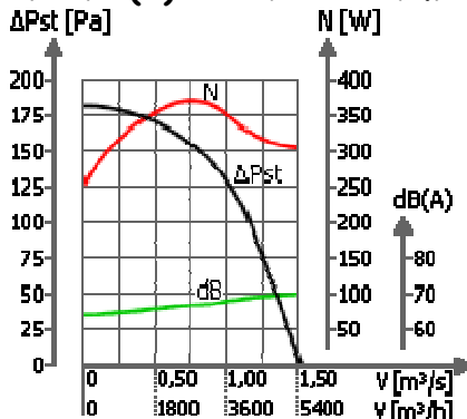
WVPKH(V)-400 /700obr/min
