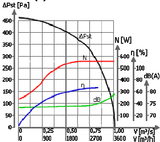
WVPKH(V)-250 /1400obr/min
