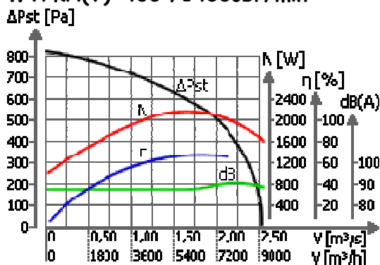
WVPKH(V)-400 /1400obr/min
