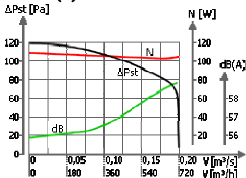
WVPKH(V)-160 /900obr/min
