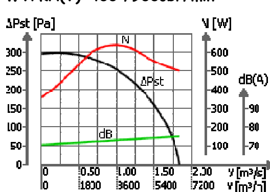
WVPKH(V)-400 /900obr/min
