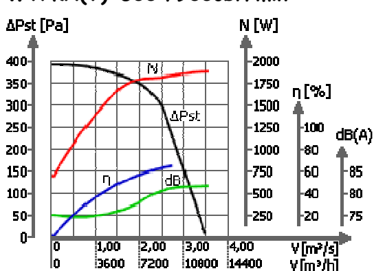
WVPKH(V)-500 /900obr/min
