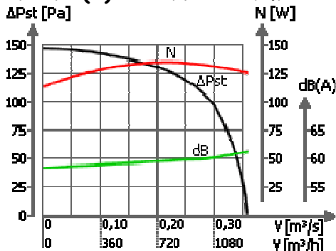
WVPKH(V)-200 /900obr/min
