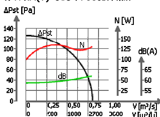
WVPKH(V)-315 /700obr/min
