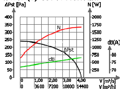
WVPKH(V)-630 /700obr/min
