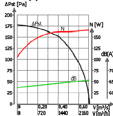
WVPKH(V)-250 /900obr/min
