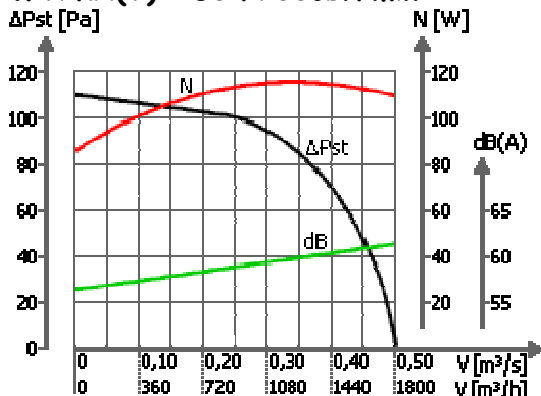
WVPKH(V)-250 /700obr/min
