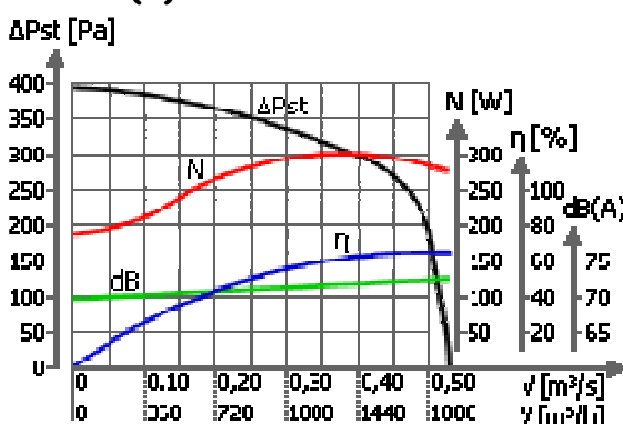
WVPKH(V)-200 /1400obr/min
