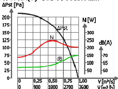
WVPKH(V)-315 /900obr/min
