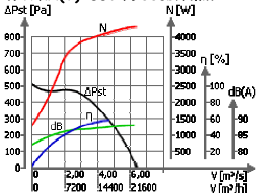
WVPKH(V)-630 /900obr/min
