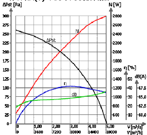
WVPKH(V)-710 /700obr/min
