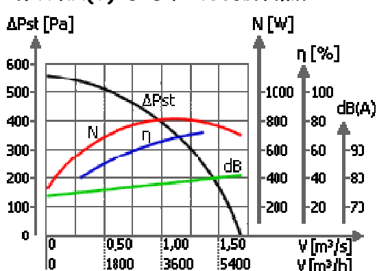
WVPKH(V)-315 /1400obr/min
