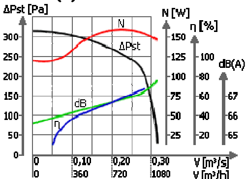
WVPKH(V)-160 /1400obr/min
