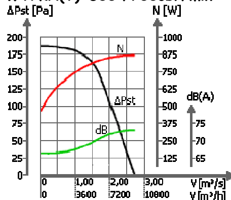
WVPKH(V)-500 /700obr/min
